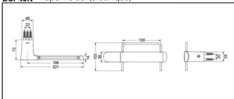
DSP43N Paper Holder (Urbanique)
